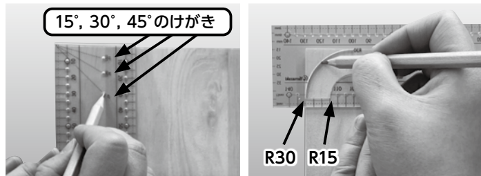
15°, 30°, 45° のけがき
