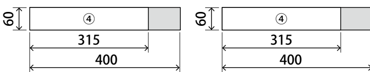
■15×60×400
