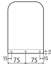
②側板 ×2
