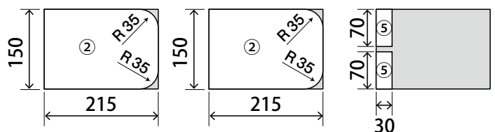
■15×150×215
