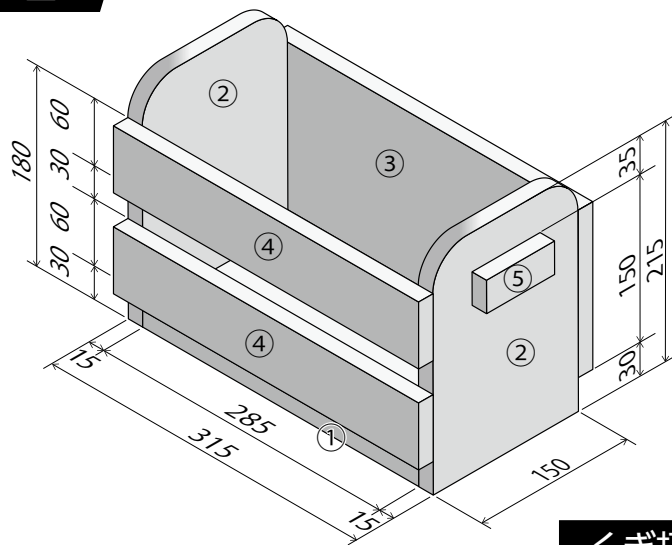
②側板 ×2
