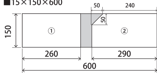
■15×150×600
