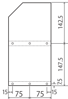
②側板 × 2
