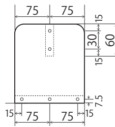
①側板 A×2
