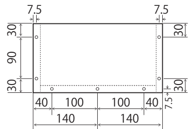
②側板 B×2
