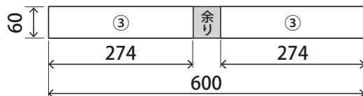
■12×60×600
