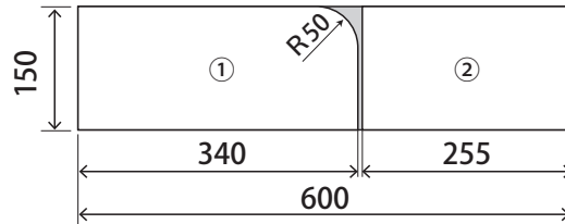
■ 15×150×600
