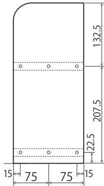
①側板 × 2
