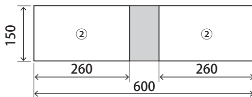
■15×150×600
