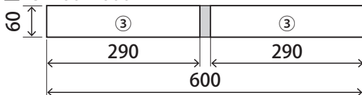
■15×60×600
