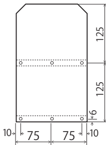
②側板 ×2
