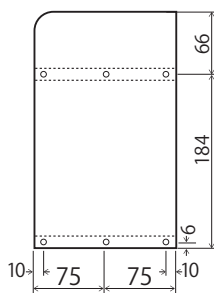
②側板 ×2
