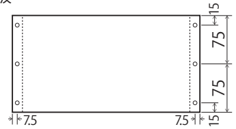
④前板 A × 2
