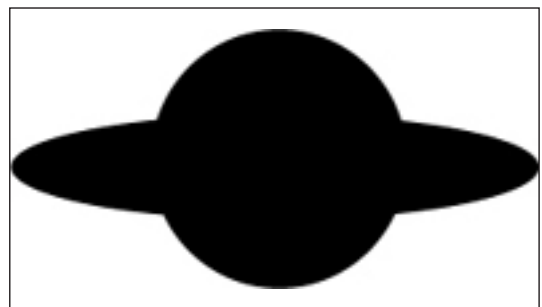
土星
