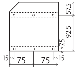
①側板 ×2
