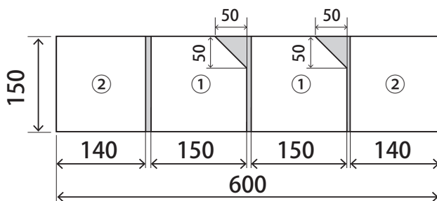
■15×150×600
