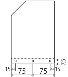
②側板 ×2
