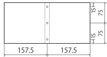
④背板 (上)
