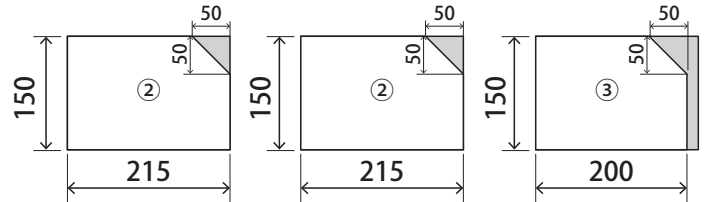
■15×150×215
