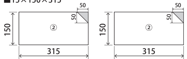
■15×150×315
