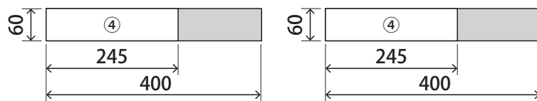
■15×60×400
