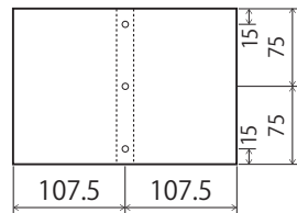
④背板 (上)
