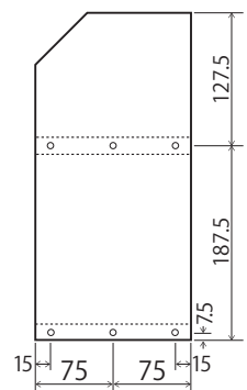
②側板 ×2
