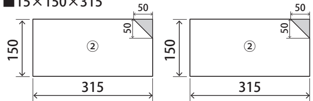
■15×150×315
