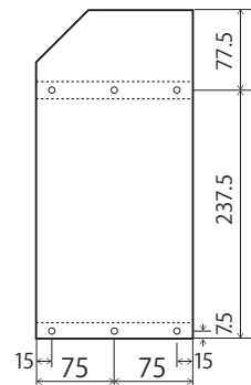
②側板 × 2
