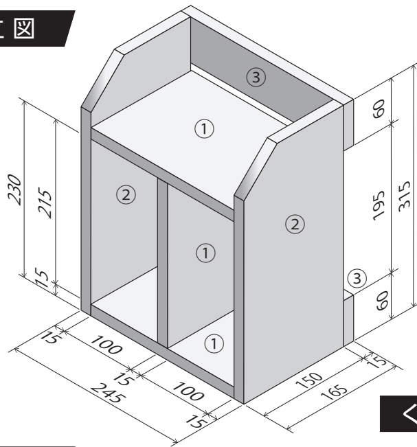
②側板 × 2
