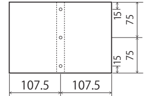
③背板 × 2
