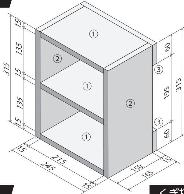
②側板 ×2
