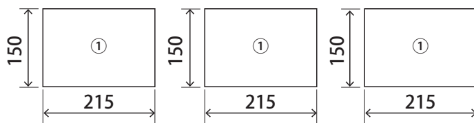
■15×150×215
