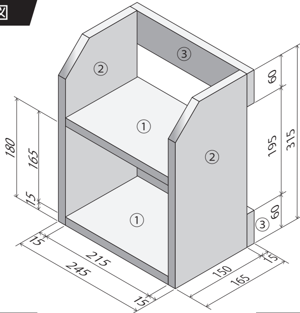
②側板 ×2
