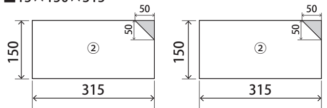
■15×150×315
