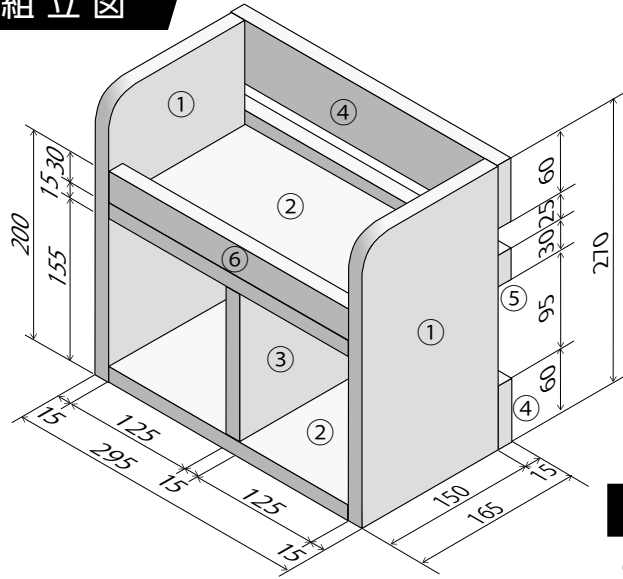
①側板
