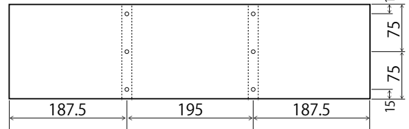
③底板
