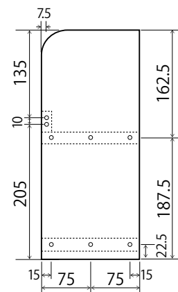
①側板 ×2
