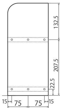
①側板 × 2
