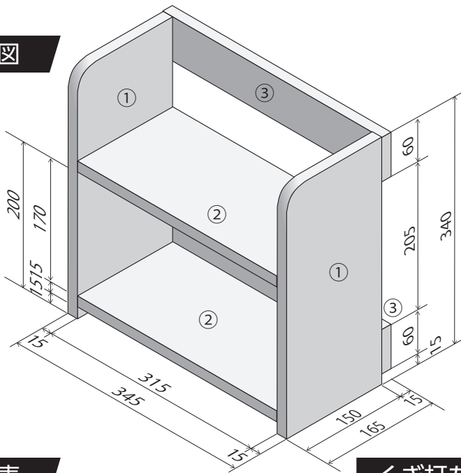
①側板 × 2
