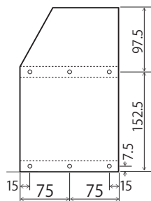
①側板 × 2
