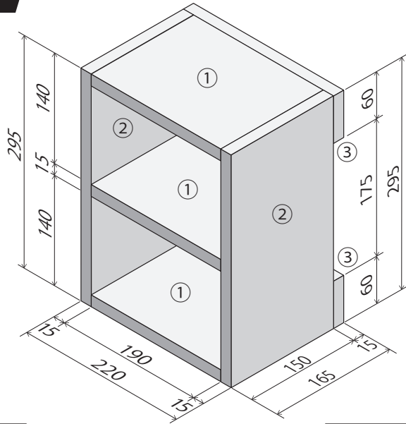
②側板 × 2
