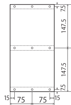
②側板 × 2
