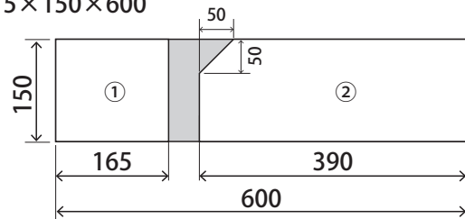
■ 15×150×600
