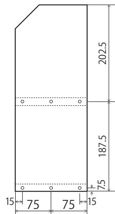
②側板 × 2
