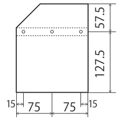
③仕切板
