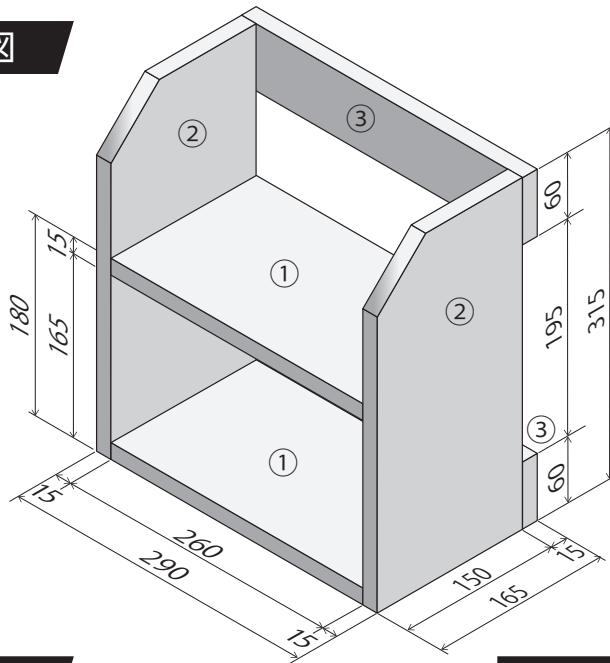
②側板 ×2
