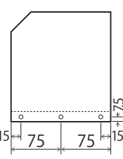
②側板 (左側)
