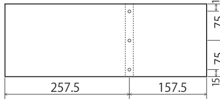
⑥背板
