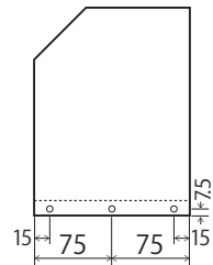
②側板 (右側)
