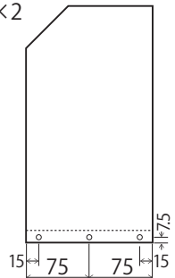
■15×150×600
