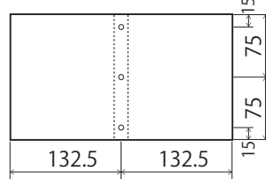
②側板 ×2
