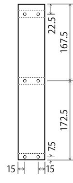
④支え板 × 2
