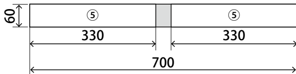
■15×60×700
