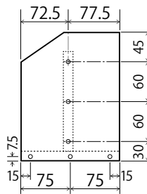
②側板 ×2
