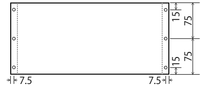
⑤前板 ×2
