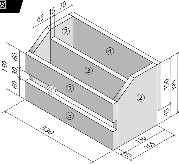
②側板 ×2
