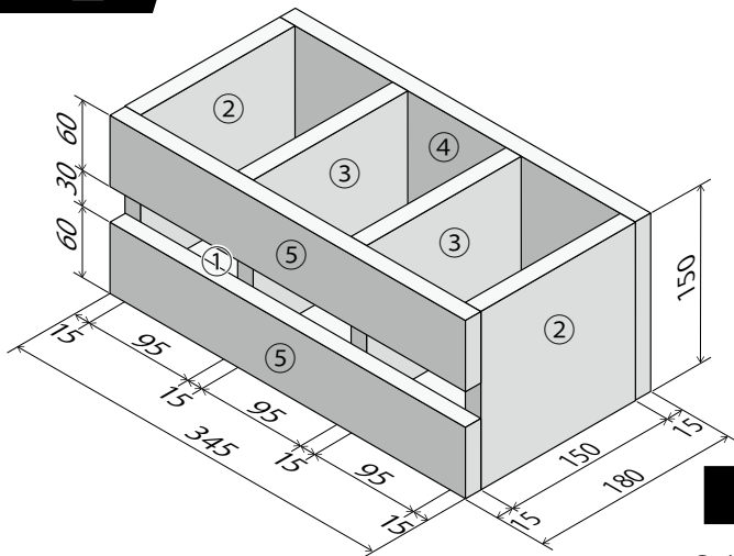
①底板
