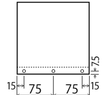
②側板 × 2
