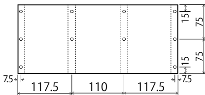
⑤前板 × 2
