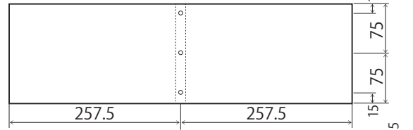
②底板
