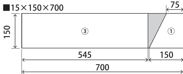
④前板
