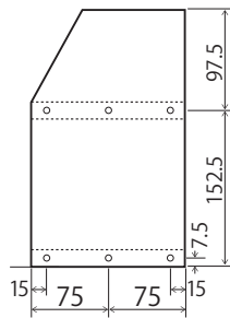
①側板 × 2
