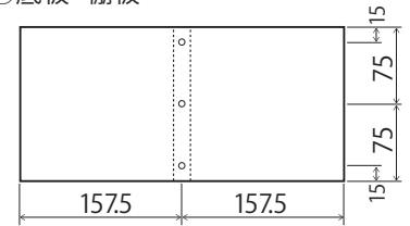
③背板 × 2
