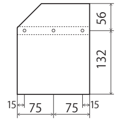
③仕切板
