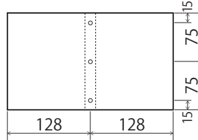
①底板 × 1
