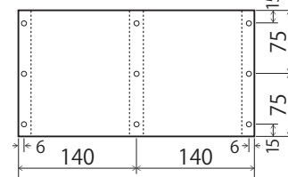
④背板 × 1
